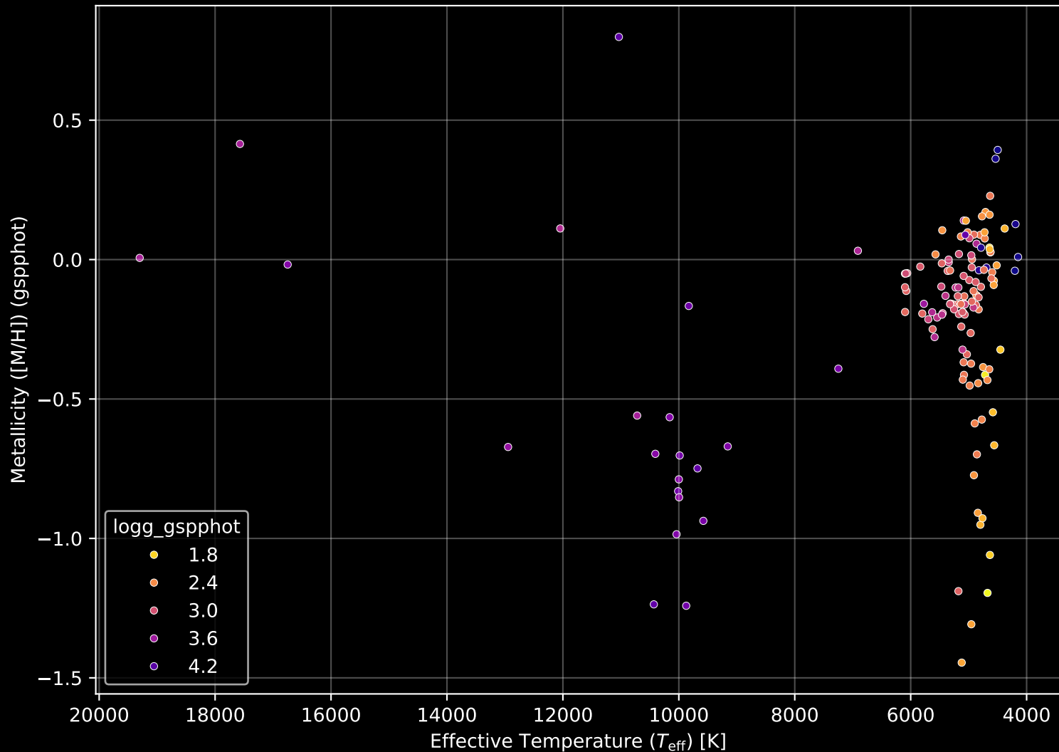
APOGEE DR17 Field: [235-06] Stellar Population Parameters (n= 144)
